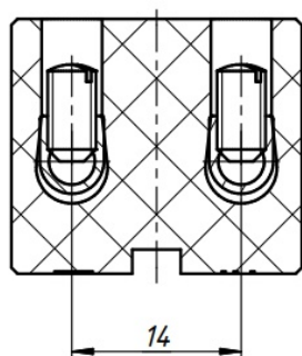
A-A (2:1)
